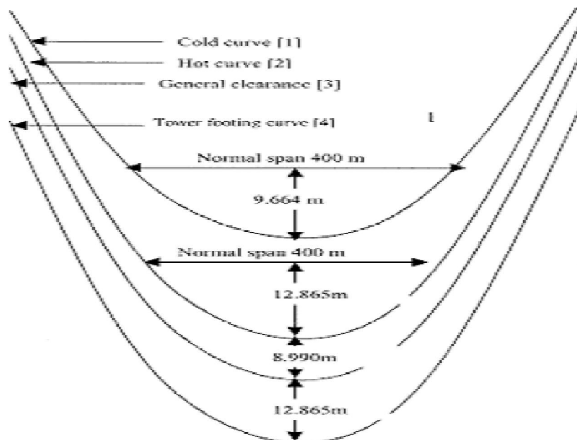
Fig 2.8- Sag Template
